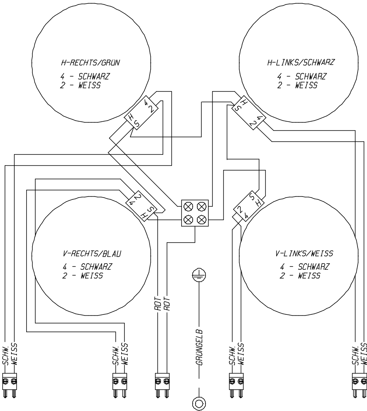
STECKERDRAUFSICHT
